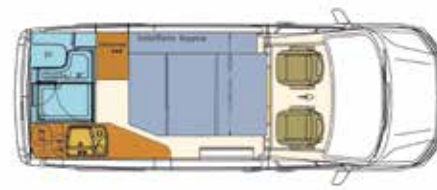
Crafter StarCamper Nachtstellung
